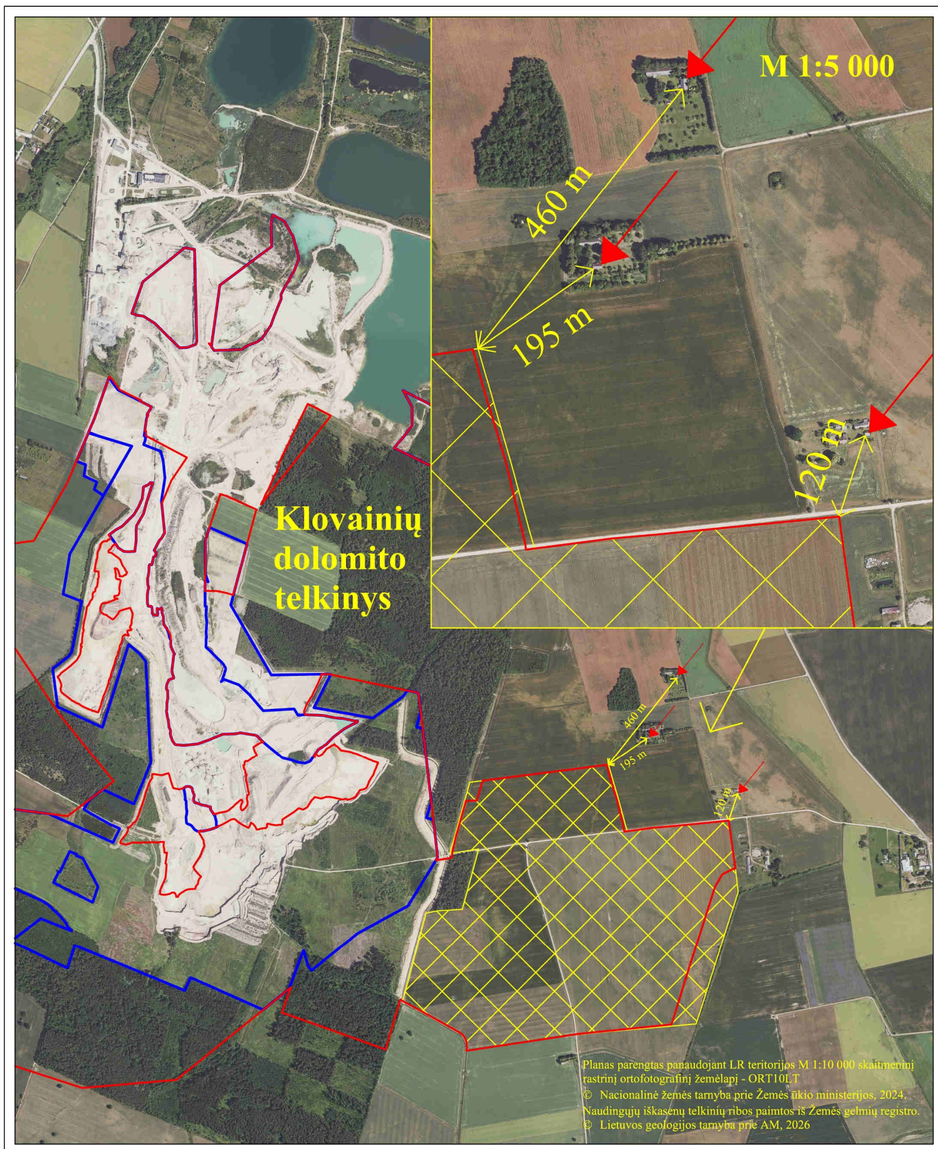
2.2 pav. Klovainių dolomito telkinio situacinis ortofotografinis planas M 1:15 000
