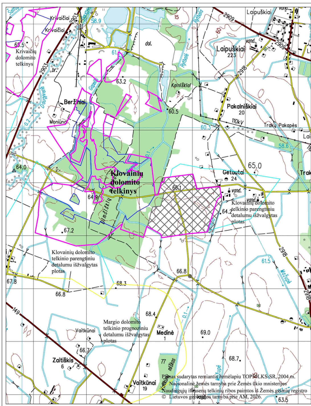
1 priedas. Klovainių dolomito telkinio apžvalginis planas M 1:25 000
